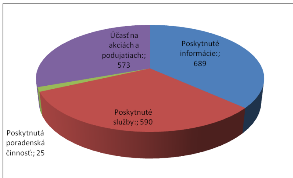
Graf č. 1: Evidencia klientov ICM Humenné v r. 2011
